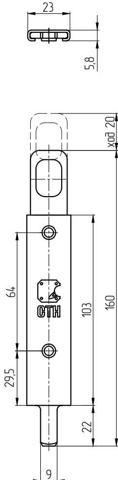
Шпингалет СТН-2403
