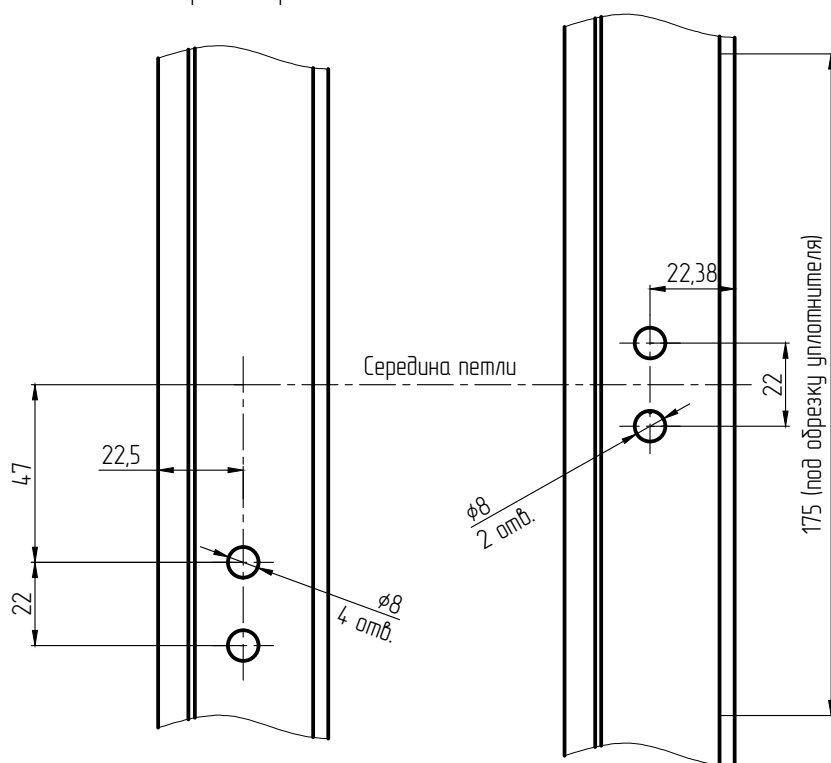
Обработка рамы
