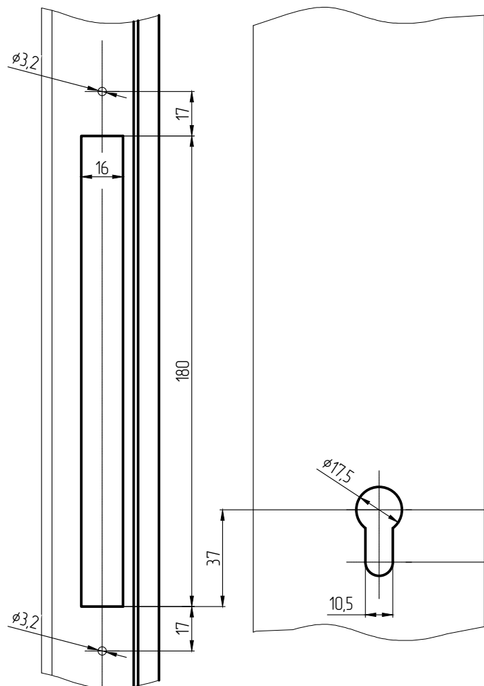
Обработка створки
